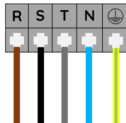
Dreiphasig
